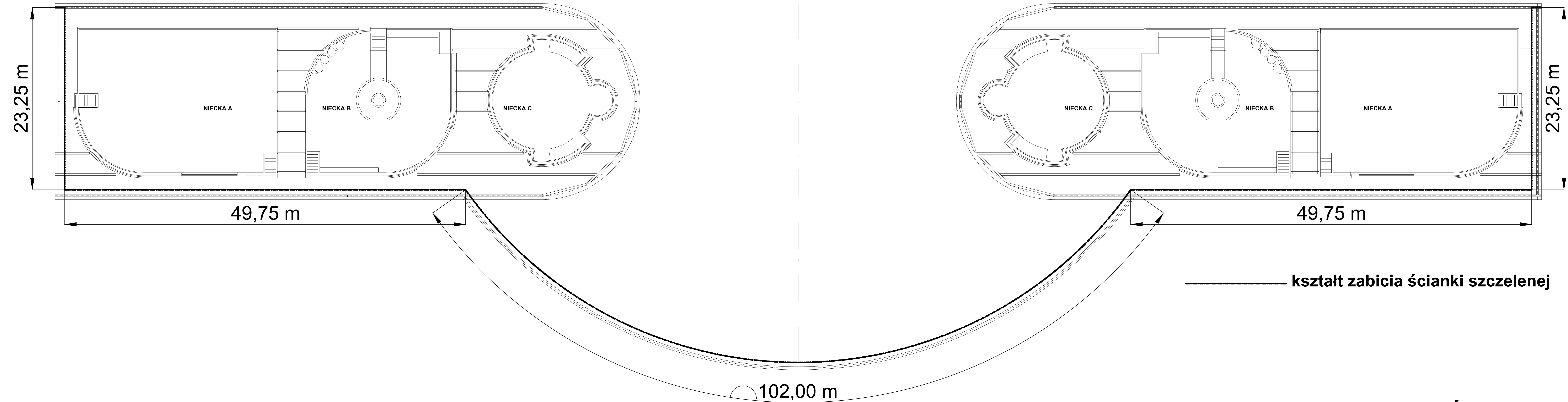
UKŁAD ZABICIA ŚCIANKI SZCZELNEJ SKALA 1:200
