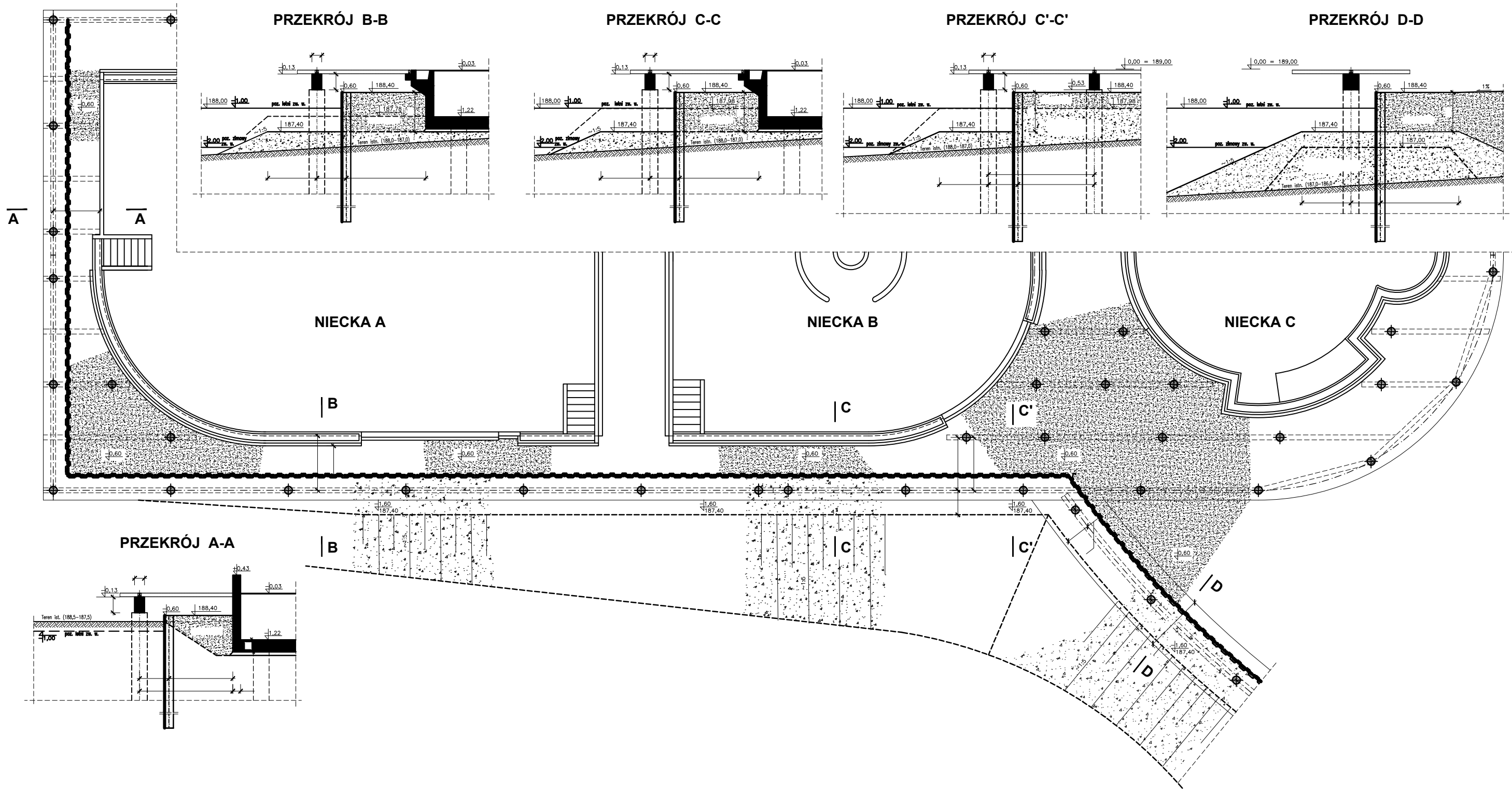
SCHEMAT ROZWIĄZANIA TECHNICZNEGO SKALA 1:200
