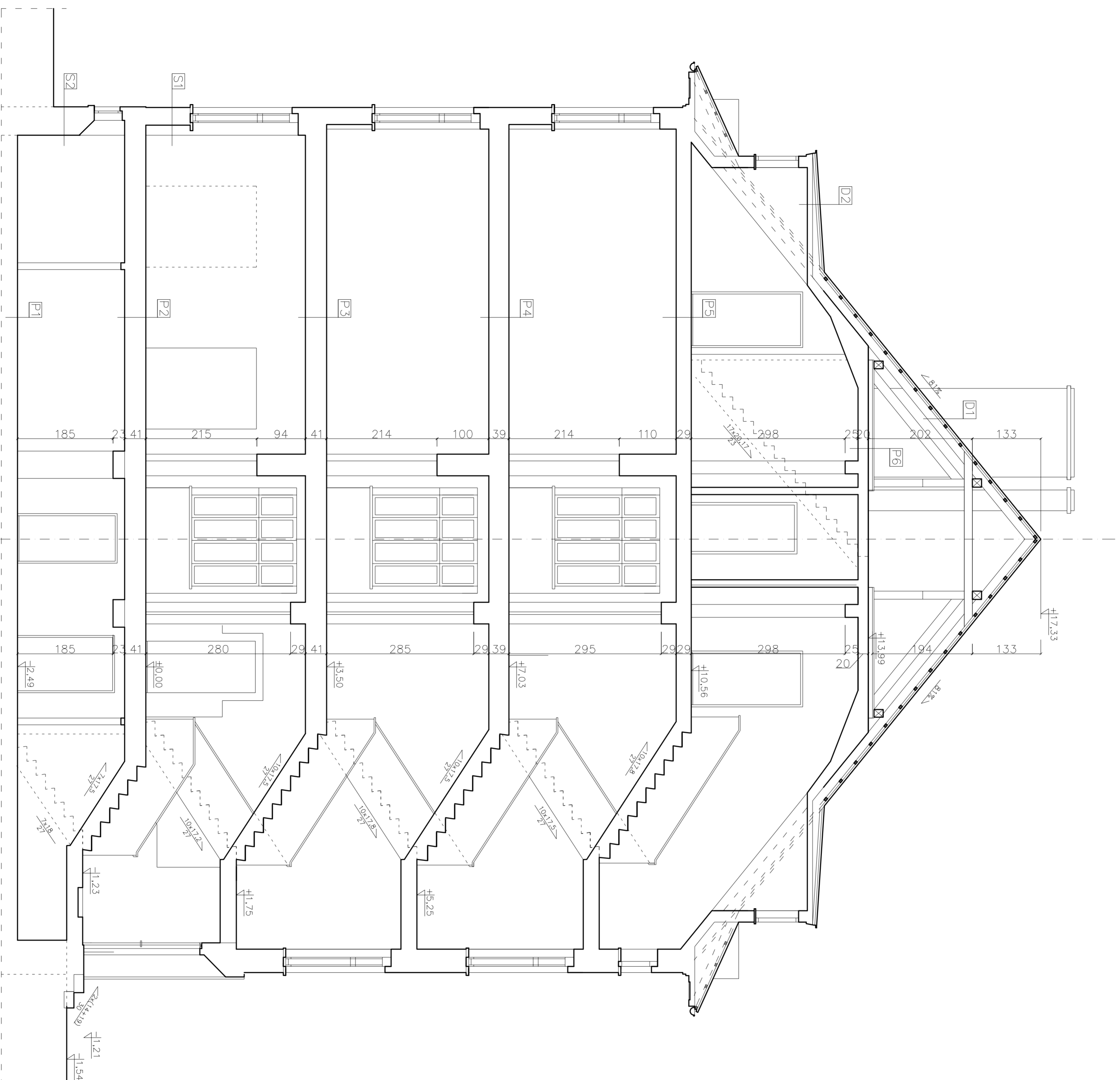
PRZEKRÓJ A-A
